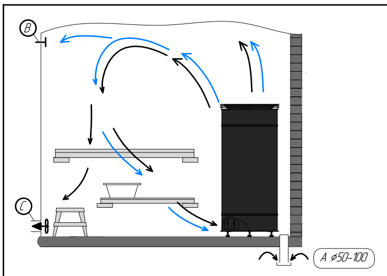
Рисунок 1. Устройство системы вентиляции в помещении:
